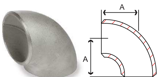
Fig. S2014E & S2016E - 90° Elbow Short Radius
