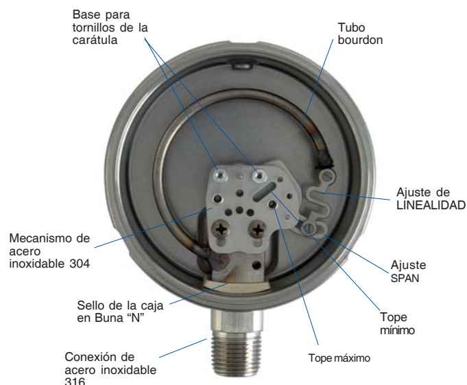
Tubos Bourdon para presiones de 1 kg/cm² hasta 60 kg/cm²
