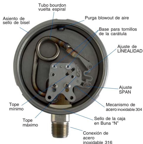
Tubos Bourdon vuelta espiral para presiones de más de 100 kg/cm²
