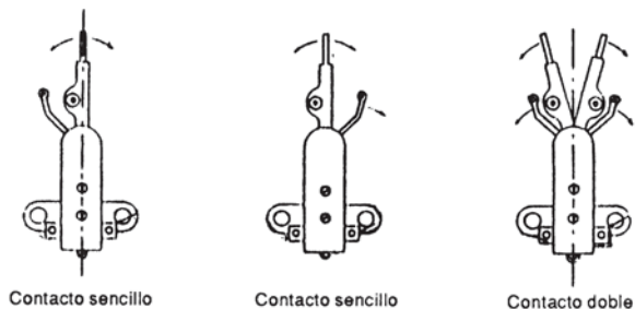
DIAGRAMA DE CONEXIONES CONTACTOS ELECTRICOS
