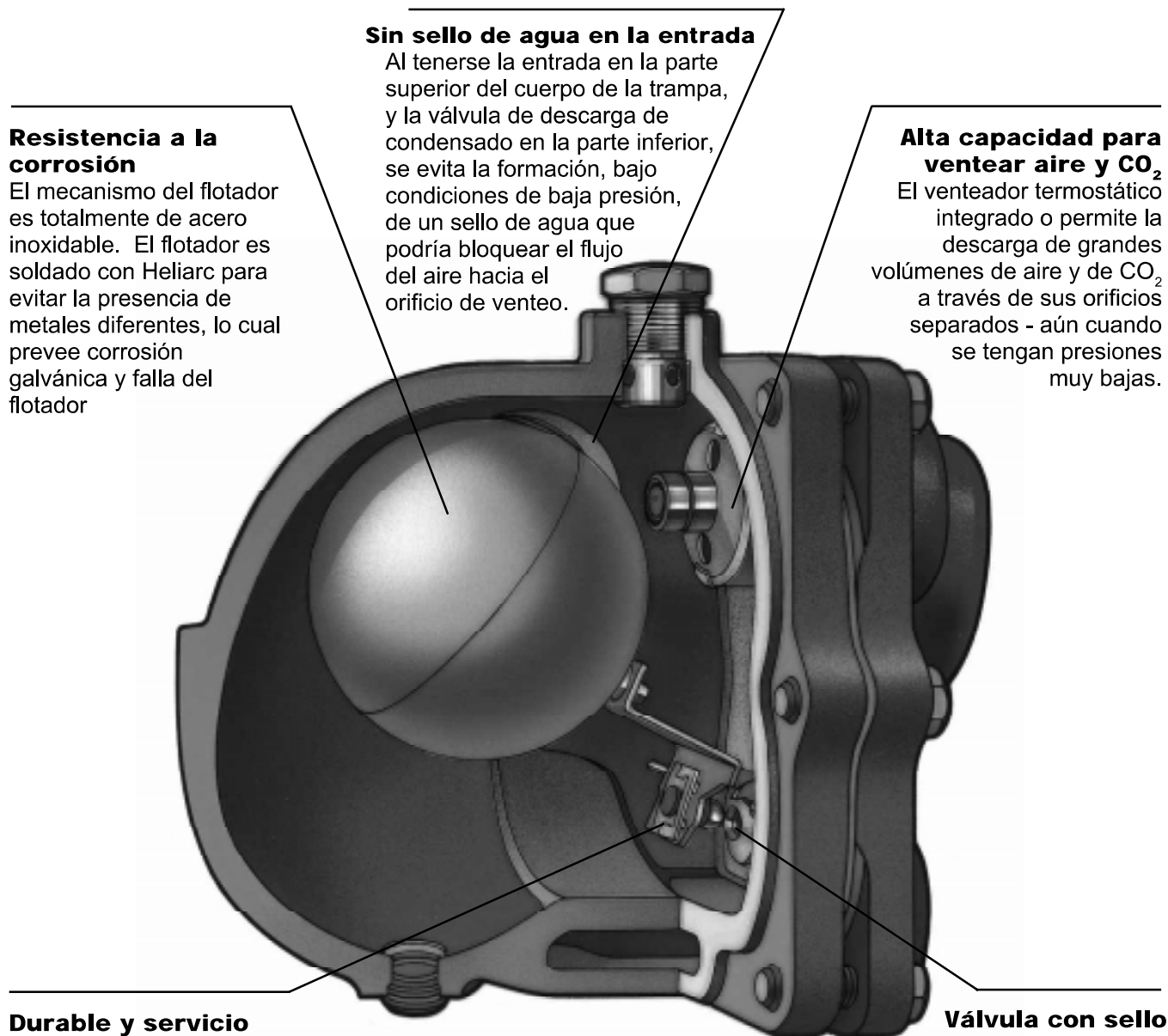
Figura 25-1. Diseño Armstrong F&T
