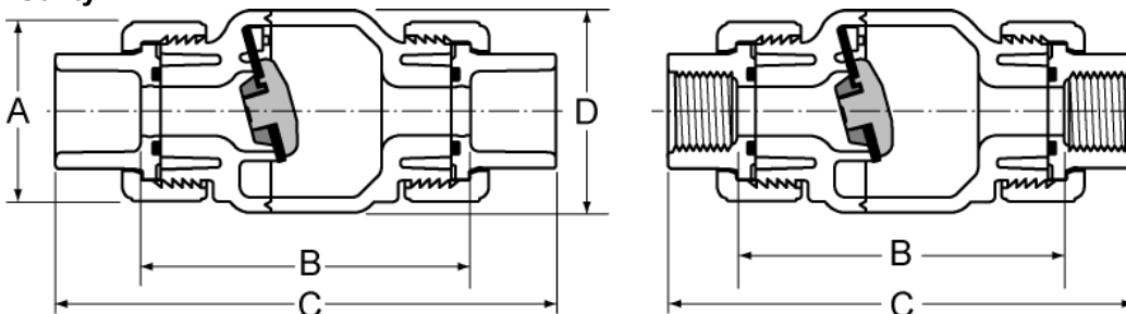
Válvulas de Retención con Resorte True Union Utility
