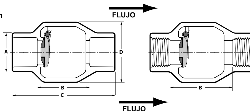
Válvula de Retención de Resorte
