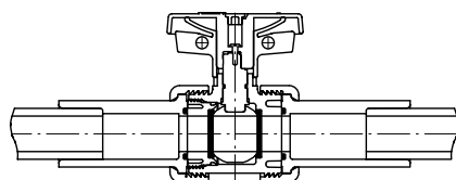
Válvula de Bola True Union 2000 Instalada con el Juego de Recambio
