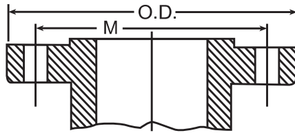
Bridas
