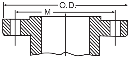
Bridas
